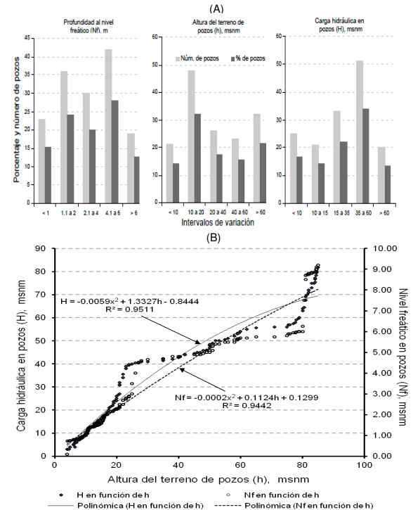
Figura 2. A. Intervalos de valores para el nivel freático (Nf), la altura del terreno (h) y la carga hidráulica (H), según el número y porcentaje de pozos. B. Tendencia y correlación numérica entre H y h, y entre Nf y h, con los respectivos modelos polinómicos (Nozagaray, 2009).
