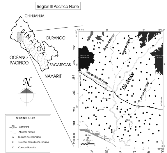
Figura 1. Localización de la Región hidrológica Pacífico Norte III y pozos en la llanura costera de la Cuenca del Río Sinaloa (Norzagaray et al. 2004).
