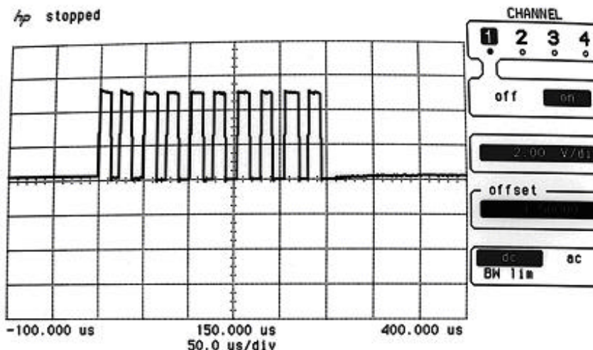
Figura 3. Tren de pulsos de transmisión producidos por STAMP BS2p
