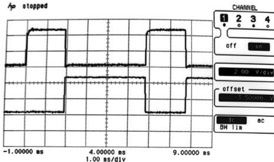
Figura 7. Señal de salida de los multivibradores monoestables para medir el tiempo de vuelo
