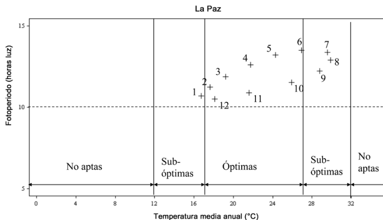
Figura 1. Aptitud climática del municipio de La Paz en función de la temperatura media mensual y fotoperiodo de 1961 – 2003. La Paz, Baja California Sur, México. Fuente: Ruiz-Corral et al. (2006).
