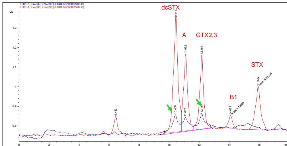
Figura 28. Cromatograma del análisis de toxinas paralizantes en hepatopáncreas de camarón durante el ensayo crónico por ingestión (día 60). Línea azul: extracto de hepatopáncreas; Línea roja: mezcla de estándares [Mix II: dcSTX, GTX2,3, B1 y SXT]. En el día 60 se pudieron detectar las toxinas paralizantes dcSTX y GTX2,3 (flechas), aún después del periodo de depuración. A= producto de oxidación secundaria de dcSTX). Oxidación: \text{H}_2\text{O}_2 [10%].
